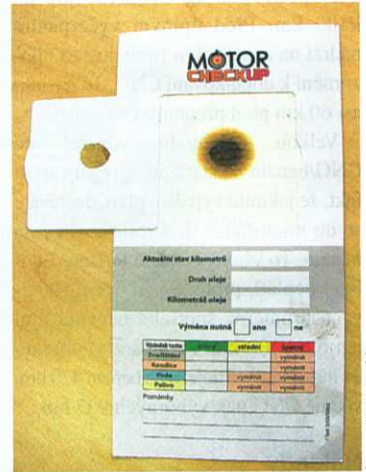
Takto vypadá kapková zkouška - kružnice u polysyntetického oleje po 10 530 km
